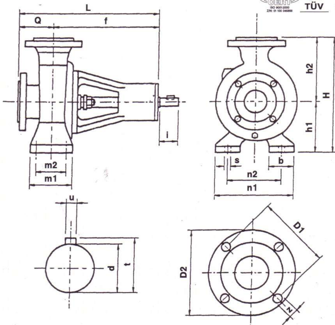
ΔΙΑΣΤΑΣΟΛΟΓΙΟ ΦΥΓΟΚΕΝΤΡΙΚΩΝ ΑΝΤΛΙΩΝ RAIN RAIN CENTRIFUGAL PUMPS DIMENSION TABLE
